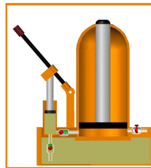
Figura 4. Accionamiento inicial del gato hidráulico.
