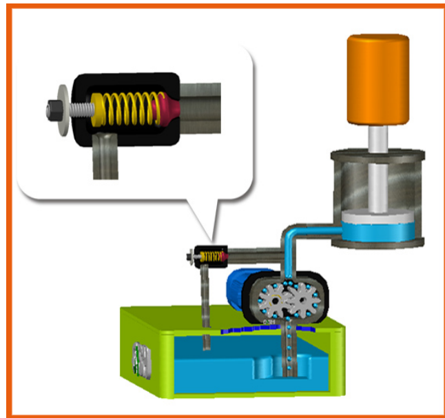
Figura 11. Acción de la válvula reguladora de presión.
