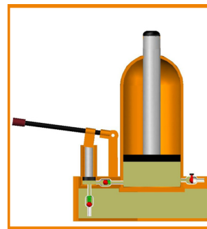
Figura 5. Fase 2 del funcionamiento del gato hidráulico.
